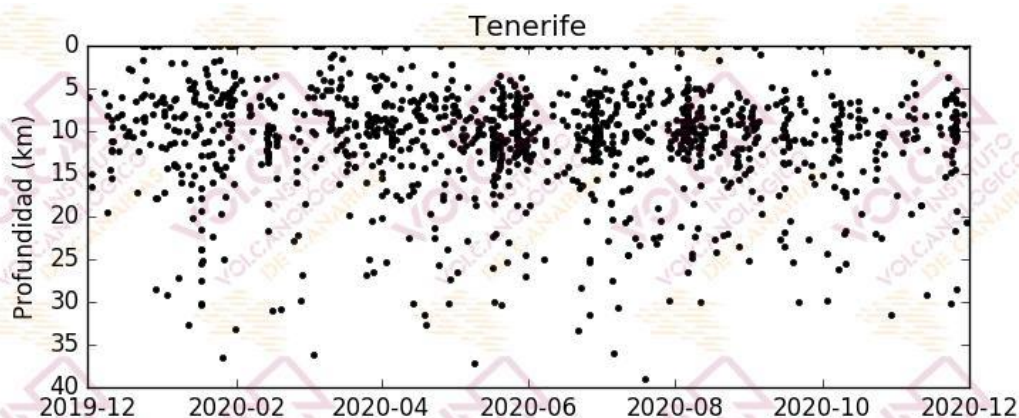
Figura 1.3 - Profundidades de los hipocentros localizados en el área de Tenerife. El gráfico superior corresponde al periodo enero 2000 - noviembre 2020, mientras que el inferior muestra el periodo diciembre 2019 - noviembre 2020. [La fuente de los datos sísmicos anteriores al 21/11/2016 es el Instituto Geográfico Nacional, IGN].
