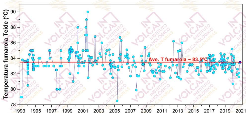
Figura 2.1 – Variaciones temporales de la temperatura registrada en las fumarolas del Teide (TEF1) desde 1993.
