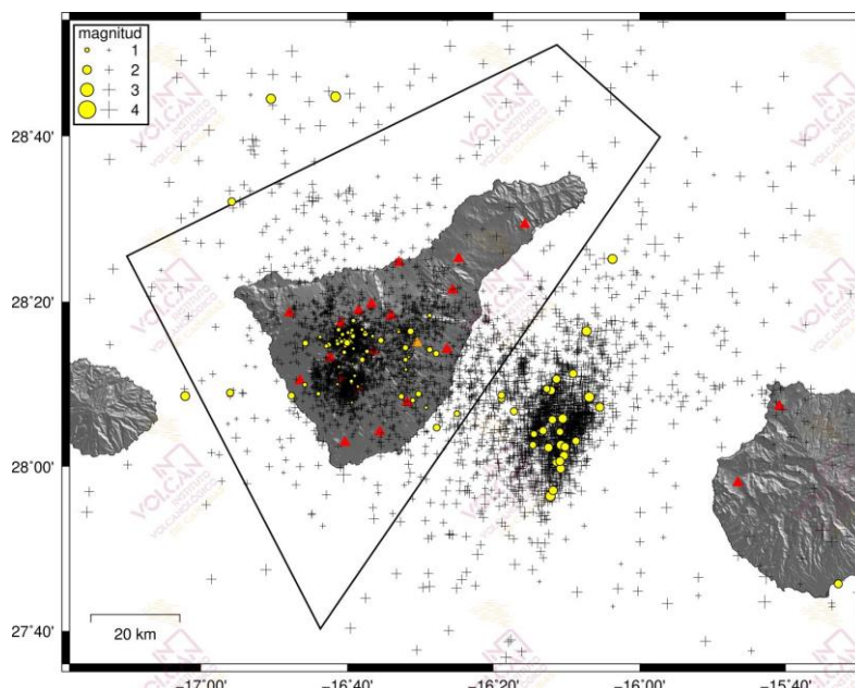
Figura 1.1 - Hipocentros de los terremotos (círculos amarillos) localizados por las estaciones de la Red Sísmica Canaria (triángulos rojos) en noviembre de 2020. Las cruces muestran los hipocentros localizados en los últimos 12 meses. El polígono negro corresponde al área de Tenerife considerada en las estadísticas sismológicas de los gráficos siguientes.
