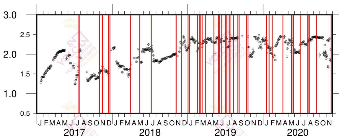
Figura 1.7 - Variaciones del parámetro b de la relación de Gutenberg-Richter durante el periodo enero 2017 – noviembre 2020. Las líneas rojas indican la ocurrencia de enjambres sísmicos.
