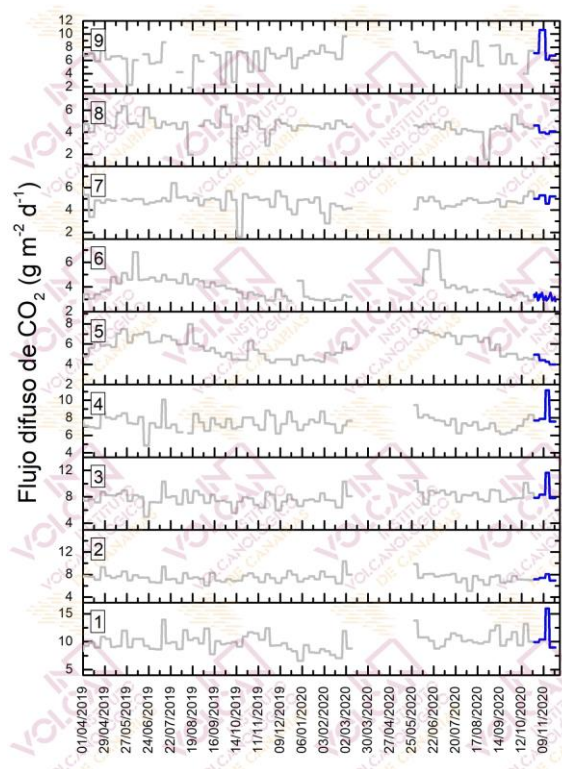
Figura 4.4 – Monitorización semanal del flujo difuso de \text{CO}_2 en la Red de Trampas Alcalinas del sistema volcánico Dorsal Noroeste de Tenerife desde abril de 2019. Los datos de noviembre de 2020 se encuentran indicados en azul oscuro.
