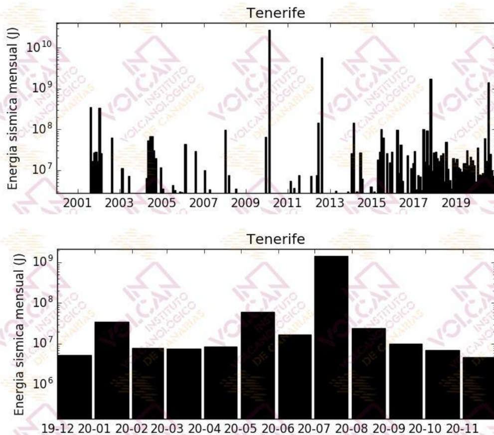
Figura 1.5 – Energía sísmica liberada por los terremotos localizados en el área de Tenerife. El histograma superior corresponde al periodo enero 2000 – noviembre 2020, mientras que el inferior muestra el periodo diciembre 2019 – noviembre 2020. [La fuente de los datos sísmicos anteriores al 21/11/2016 es el Instituto Geográfico Nacional].
