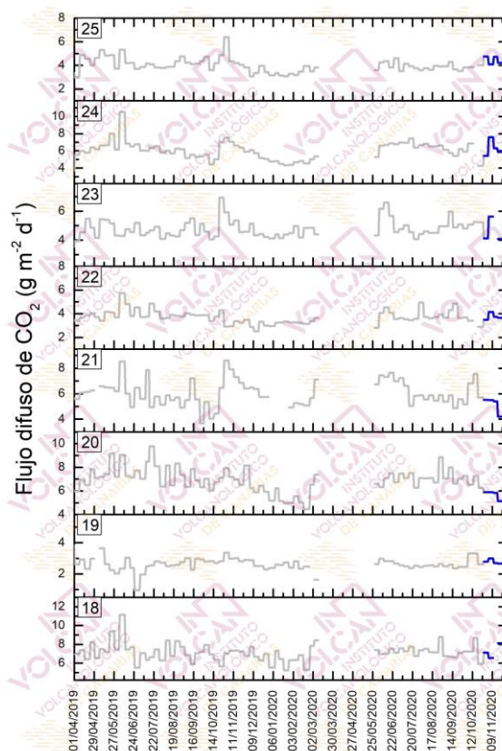
Figura 4.7 – Monitorización semanal del flujo difuso de \text{CO}_2 en la Red de Trampas Alcalinas de la Caldera de Las Cañadas desde abril de 2019. Los datos de noviembre de 2020 se encuentran indicados en azul oscuro.
