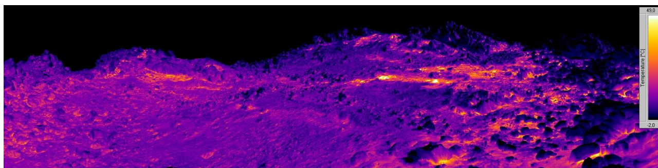
Figura 2.4 – Imagen térmica del cráter del Teide obtenida con cámara la térmica FLIR T660 en noviembre 2020.
