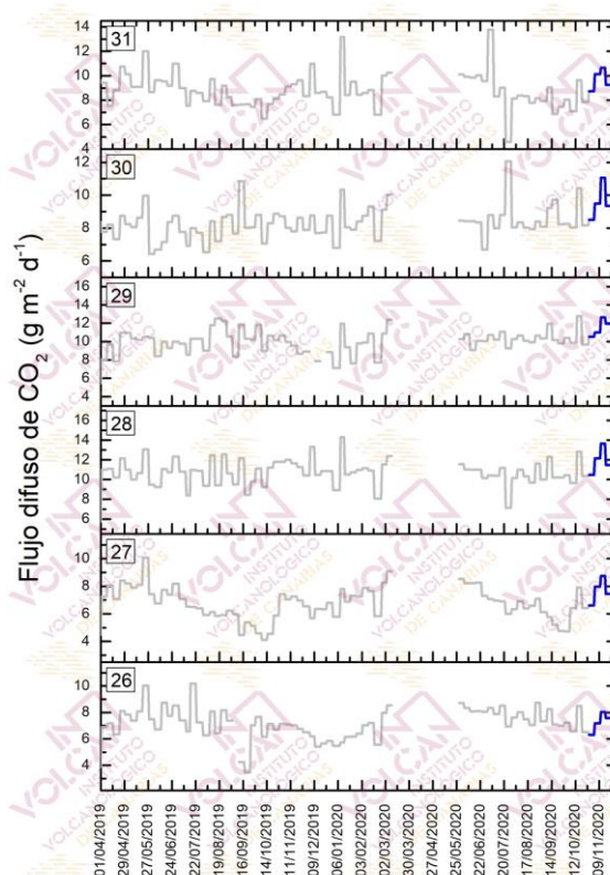
Figura 4.5 – Monitorización semanal del flujo difuso de \text{CO}_2 en la Red de Trampas Alcalinas del sistema volcánico Dorsal Noreste de Tenerife desde abril de 2019. Los datos de noviembre de 2020 se encuentran indicados en azul oscuro.
