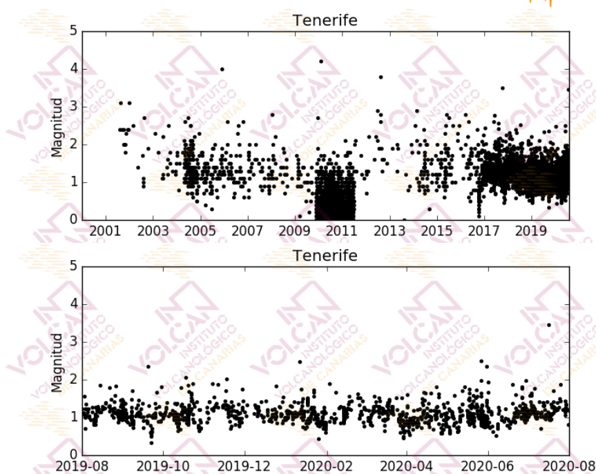
Figura 1.4 - Magnitudes de los terremotos localizados en el área de Tenerife. El gráfico superior corresponde al periodo enero 2000 – julio 2020, mientras que el inferior muestra el periodo agosto 2019 – julio 2020. [La fuente de los datos sísmicos anteriores al 21/11/2016 es el Instituto Geográfico Nacional, IGN].
