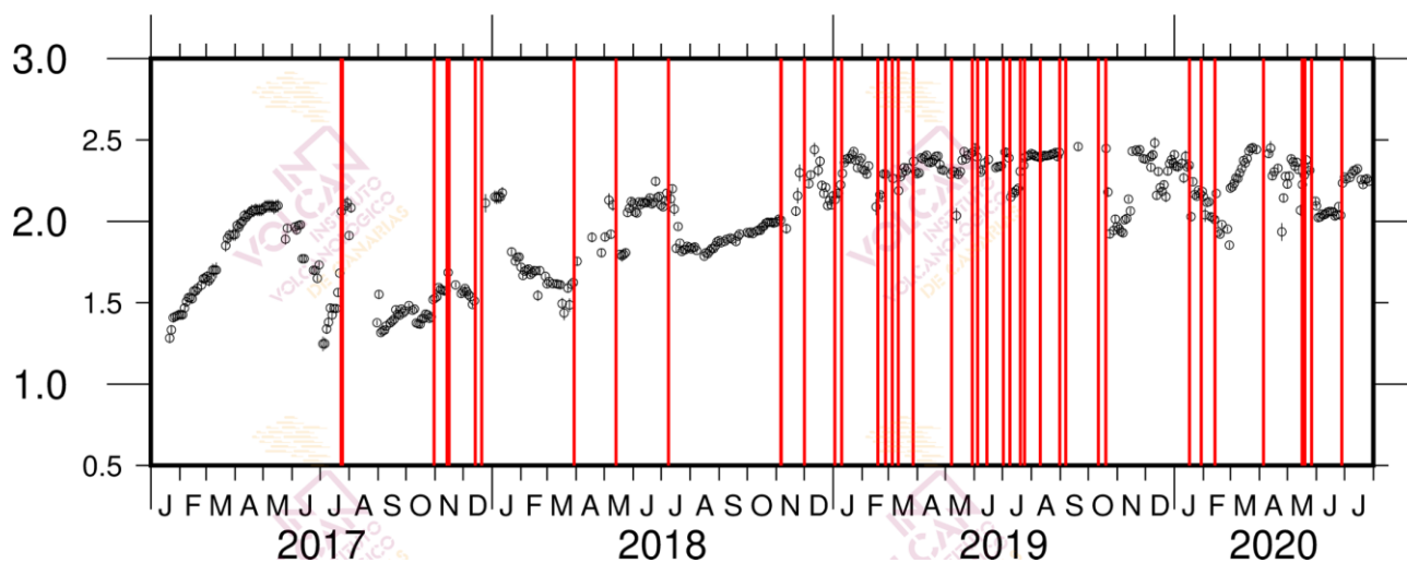
Figura 1.7 - Variaciones del parámetro b de la relación de Gutenberg-Richter durante el periodo enero 2017 – julio 2020. Las líneas rojas indican la ocurrencia de enjambres sísmicos.
