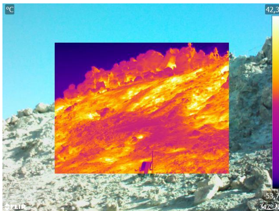
Figura 2.3. Zona del cráter del Teide seleccionada para el seguimiento termográfico con la cámara térmica e imagen térmica obtenida con cámara la térmica FLIR T660 en el mes de julio de 2020.
