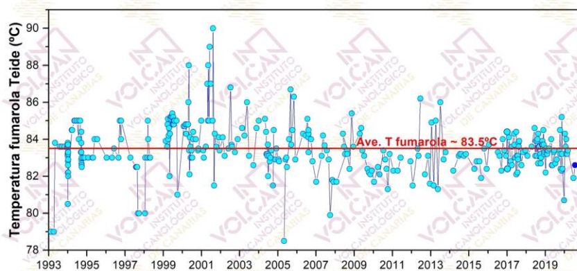
Figura 2.1 – Variaciones temporales de la temperatura registrada en las fumarolas del Teide (TEF1) desde 1993. Los datos de julio de 2020 se encuentran indicados en azul oscuro.
