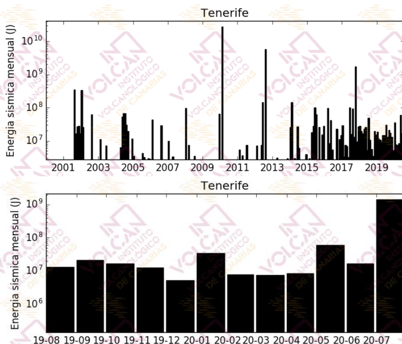
Figura 1.5 – Energía sísmica liberada por los terremotos localizados en el área de Tenerife. El histograma superior corresponde al periodo enero 2000 – julio 2020, mientras que el inferior muestra el periodo agosto 2019 – julio 2020. [La fuente de los datos sísmicos anteriores al 21/11/2016 es el Instituto Geográfico Nacional].
