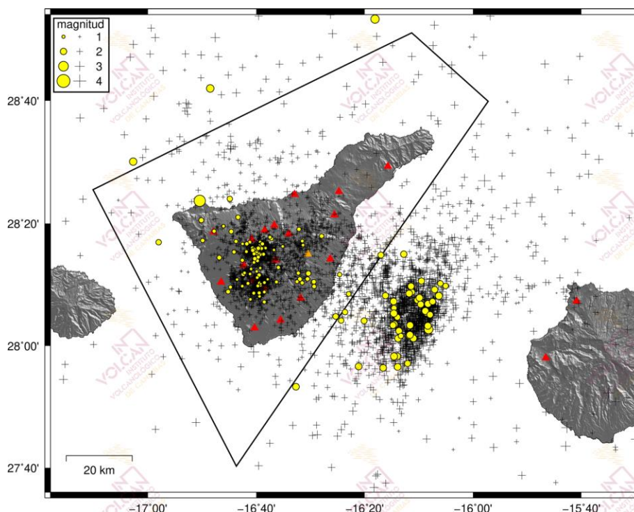
Figura 1.1 - Hipocentros de los terremotos (círculos amarillos) localizados por las estaciones de la Red Sísmica Canaria (triángulos rojos) en julio de 2020. Las cruces muestran los hipocentros localizados en los últimos 12 meses. El polígono negro corresponde al área de Tenerife considerada en las estadísticas sismológicas de los gráficos siguientes.
