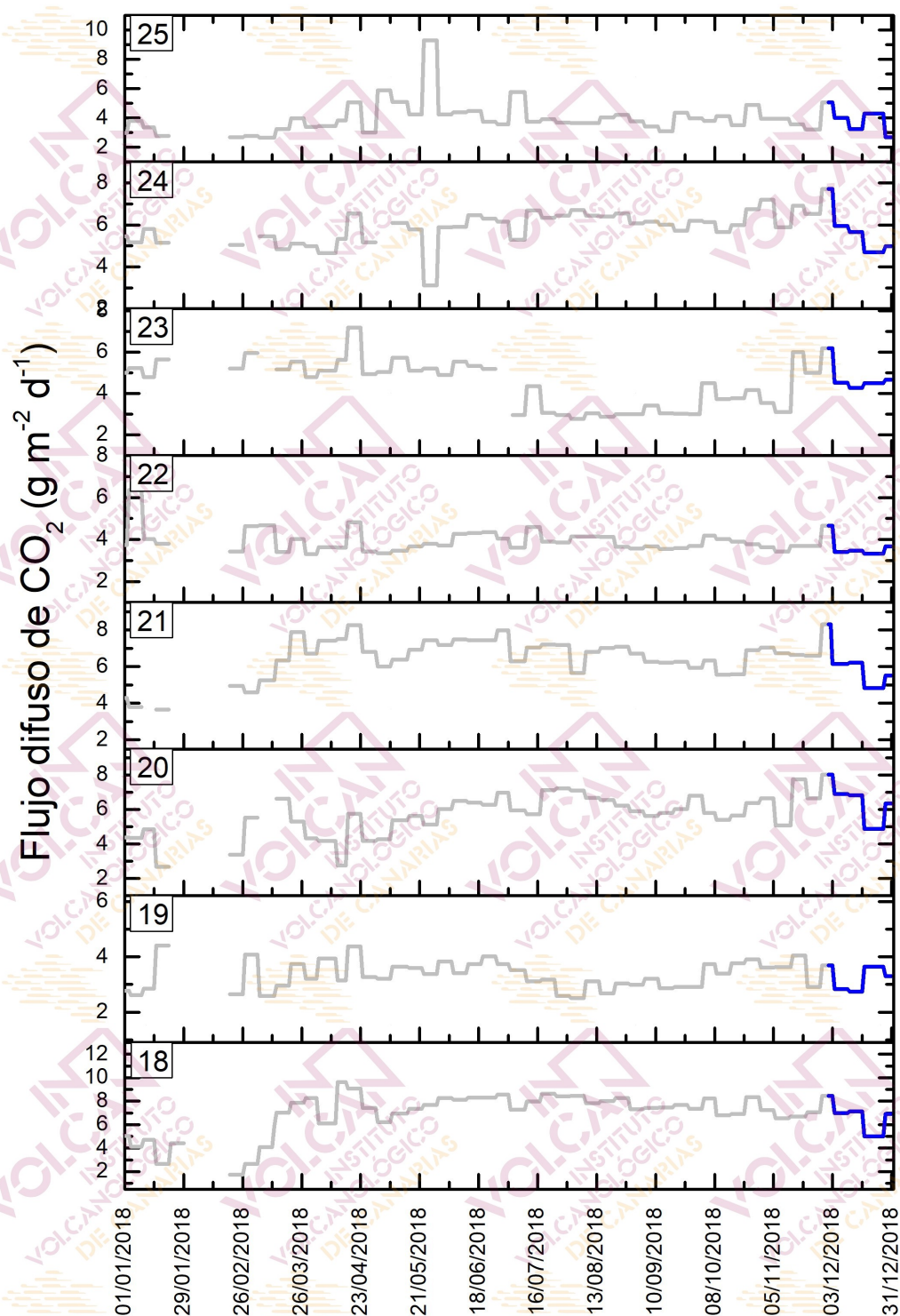
Figura 4.7 – Monitorización semanal del flujo difuso de CO 2 en la Red de Trampas Alcalinas de la Caldera de Las Cañadas durante los últimos 12 meses. Los datos de diciembre de 2018 se encuentran marcados en azul oscuro.
