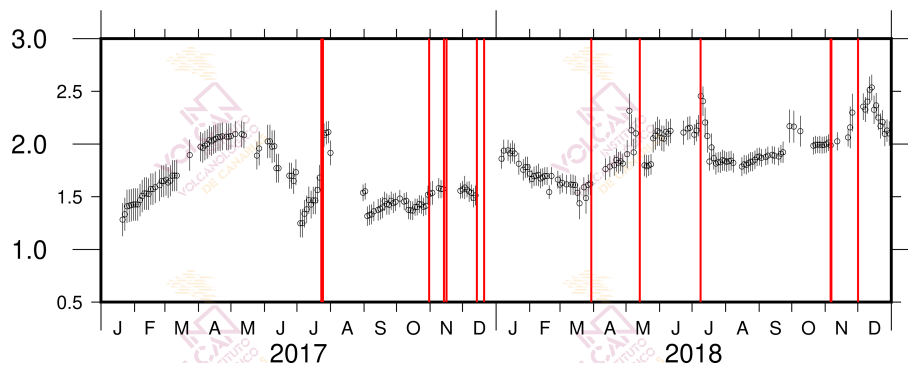
Figura 1.7 - Variaciones del parámetro b de la relación de Gutenberg-Richter desde enero 2017 hasta diciembre 2018. Las líneas rojas indican la ocurrencia de enjambres sísmicos.
