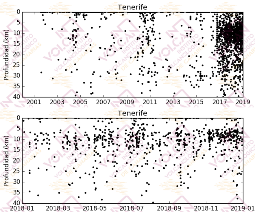
Figura 1.3 - Profundidades de los hipocentros localizados en el área de Tenerife. El gráfico superior corresponde al periodo enero 2000- diciembre 2018, mientras que el inferior muestra el periodo enero 2018- diciembre 2018. [La fuente de los datos sísmicos anteriores al 21/11/2016 es el Instituto Geográfico Nacional, IGN].
