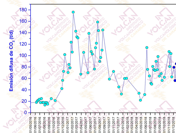
Figura 4.3 – Variaciones temporales de la emisión difusa de dióxido de carbono ( \text{CO}_2 ) en el cráter del Teide desde el 1 de junio de 2016. Los datos de diciembre de 2018 se encuentran marcados en azul oscuro.
