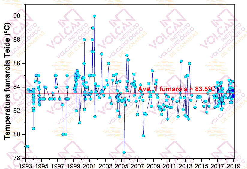
Figura 2.1 – Variaciones temporales de la temperatura registrada en las fumarolas del Teide (TEF1) desde 1993. Los datos de diciembre de 2018 se encuentran marcados en azul oscuro.
