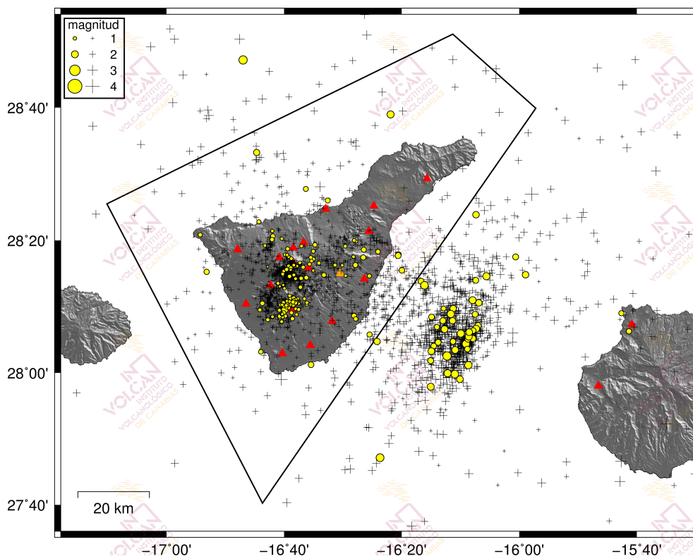
Figura 1.1 - Hipocentros de los terremotos (círculos amarillos) localizados por las estaciones de la Red Sísmica Canaria (triángulos rojos) en diciembre de 2018. Las cruces muestran los hipocentros localizados en los últimos 12 meses. El polígono negro corresponde al área de Tenerife considerada en las estadísticas sismológicas de los gráficos siguientes.
