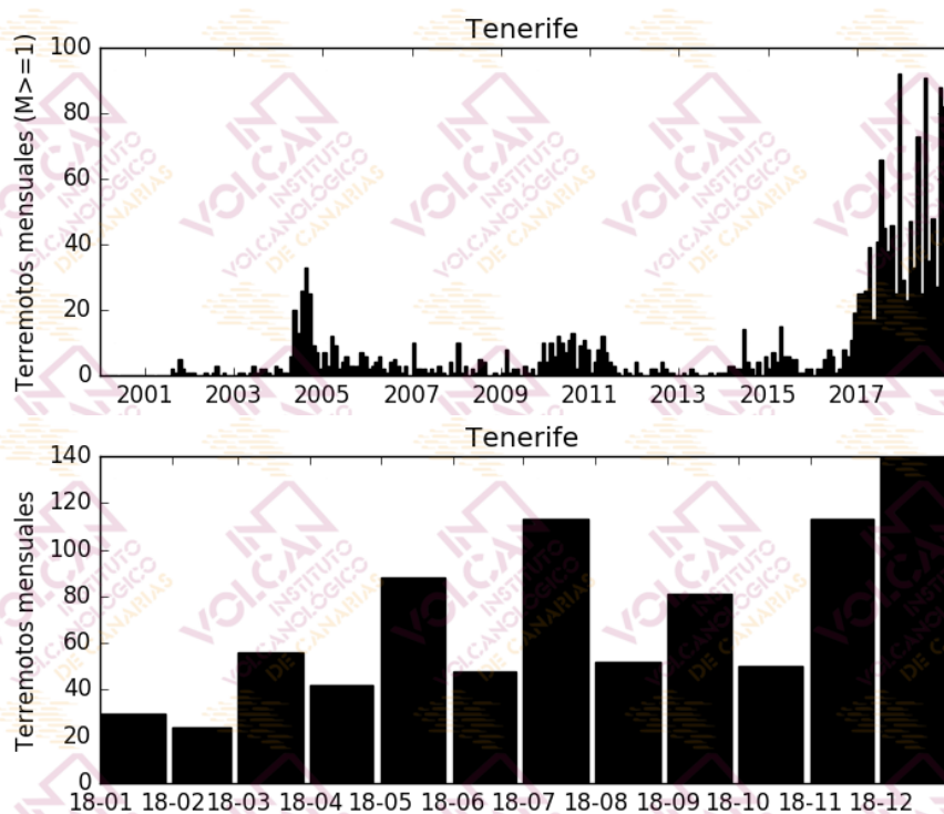
Figura 1.2 - Número de terremotos mensuales en Tenerife. El histograma superior corresponde al periodo enero 2000- diciembre 2018 para terremotos con M \geq 1 , mientras que el inferior muestra el periodo enero 2018- diciembre 2018 para todas las magnitudes. [La fuente de los datos sísmicos anteriores al 21/11/2016 es el Instituto Geográfico Nacional, IGN].
