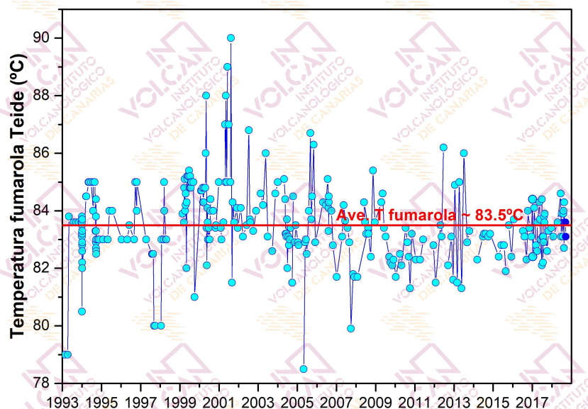
Figura 2.1 – Variaciones temporales de la temperatura registrada en la fumarola del Teide (TEF1) desde 1993. Los datos de septiembre de 2018 se encuentran marcados en azul oscuro.
