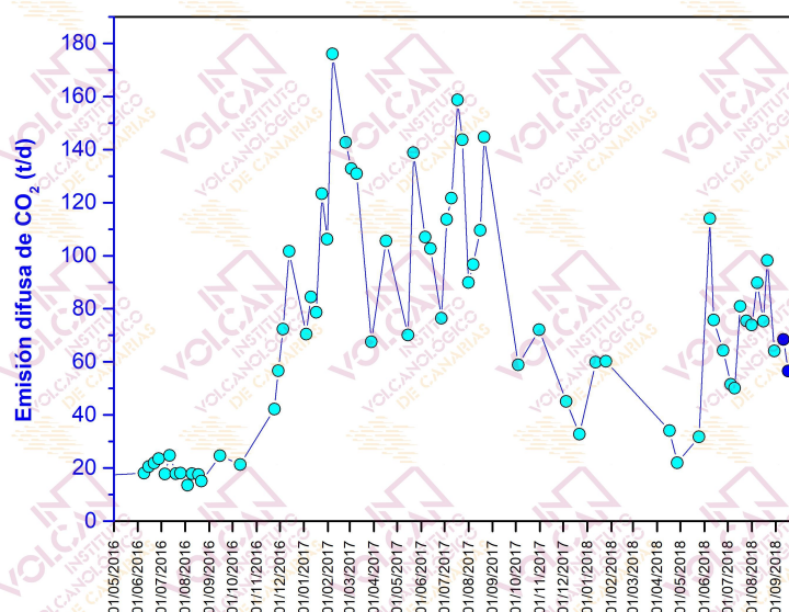
Figura 4.3 – Variaciones temporales de la emisión difusa de dióxido de carbono ( \text{CO}_2 ) en el cráter del Teide desde el 1 de junio de 2016. Los datos de septiembre de 2018 se encuentran marcados en azul oscuro.
