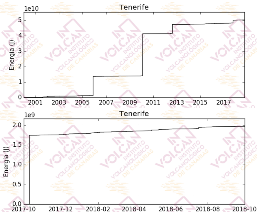
Figura 1.6 - Curva de energía sísmica acumulada por los terremotos localizados en el área de Tenerife. El gráfico superior corresponde al periodo enero 2000-septiembre 2018, mientras que el inferior muestra el periodo octubre 2017-septiembre 2018. [La fuente de los datos sísmicos anteriores al 21/11/2016 es el Instituto Geográfico Nacional, IGN].
