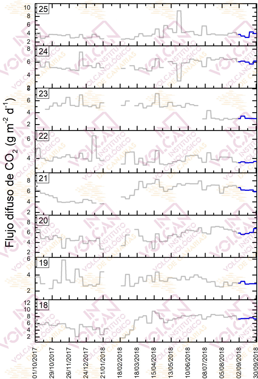
Figura 4.7 – Monitorización semanal del flujo difuso de CO 2 en la Red de Trampas Alcalinas de la Caldera de Las Cañadas durante los últimos 12 meses. Los datos de septiembre de 2018 se encuentran marcados en azul oscuro.
