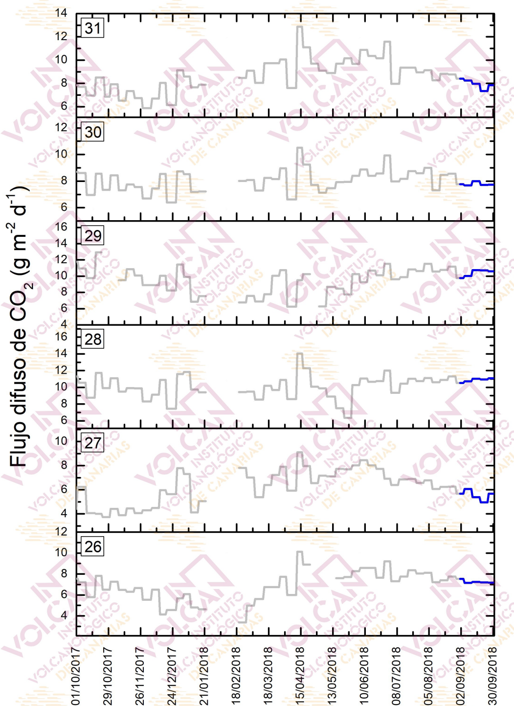
Figura 4.5 – Monitorización semanal del flujo difuso de CO 2 en la Red de Trampas Alcalinas del sistema volcánico Dorsal Noreste de Tenerife durante los últimos 12 meses. Los datos de septiembre de 2018 se encuentran marcados en azul oscuro.
