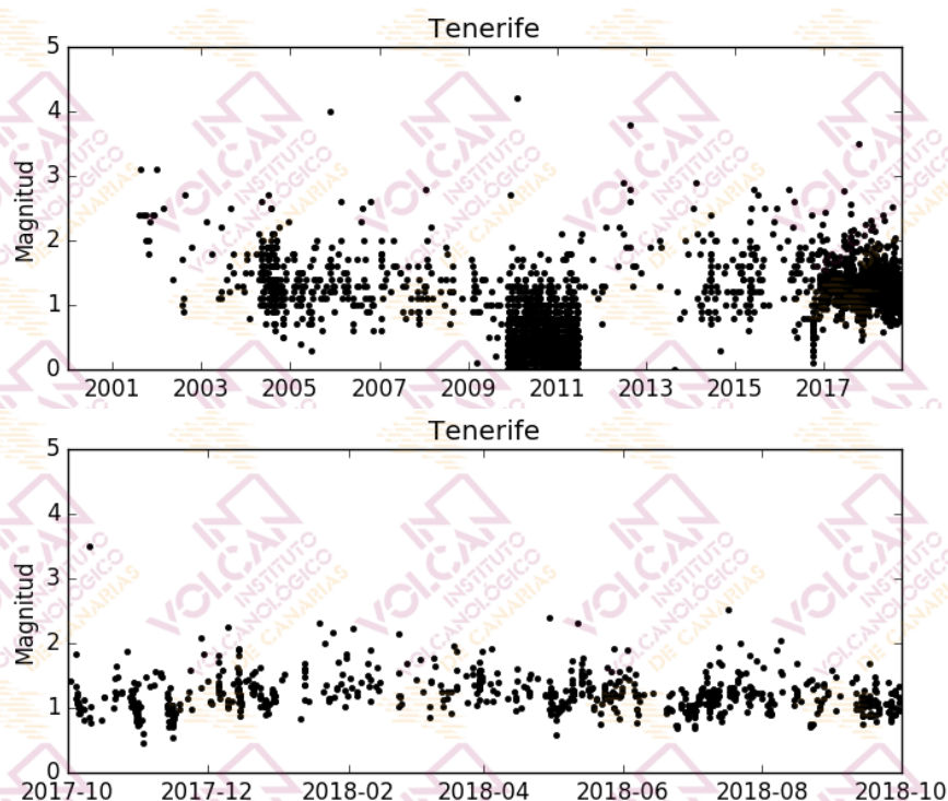
Figura 1.4 - Magnitudes de los terremotos localizados en el área de Tenerife. El gráfico superior corresponde al periodo enero 2000-septiembre 2018, mientras que el inferior muestra el periodo octubre 2017-septiembre 2018. [La fuente de los datos sísmicos anteriores al 21/11/2016 es el Instituto Geográfico Nacional, IGN].
