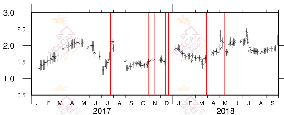
Figura 1.7 - Variaciones del parámetro b de la relación de Gutenberg-Richter desde enero 2017 hasta septiembre 2018. Las líneas rojas indican la ocurrencia de enjambres sísmicos.
