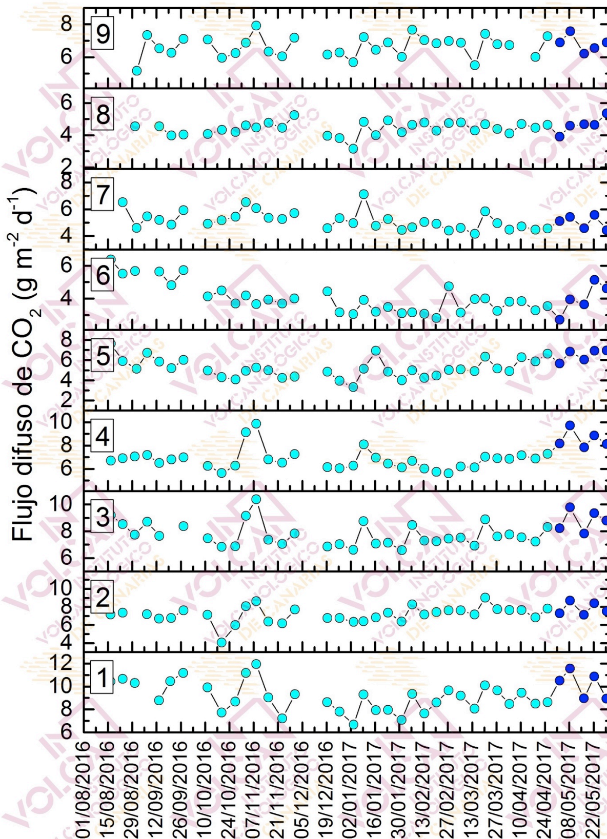
Figura 4.4 – Monitorización semanal del flujo difuso de CO 2 en la Red de Trampas Alcalinas del sistema volcánico Dorsal Noroeste de Tenerife desde agosto de 2016. Los datos de mayo de 2017 se encuentran marcados en azul oscuro.
