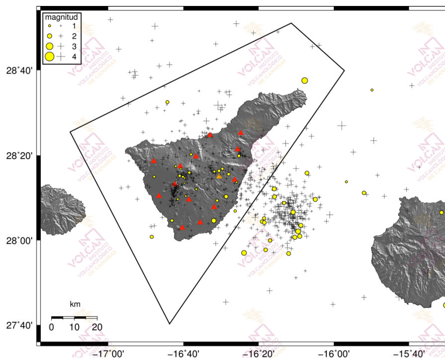
Figura 1.1 - Hipocentros de los terremotos localizados por la Red Sísmica Canaria (triángulos rojos) en mayo de 2017 (círculos amarillos). Las cruces muestran los hipocentros localizados en los últimos 12 meses. El polígono negro corresponde al área de Tenerife considerada para las estadísticas sismológicas en los gráficos siguientes. [La fuente de los datos sísmicos anteriores al 21/11/2016 es el Instituto Geográfico Nacional, IGN].
