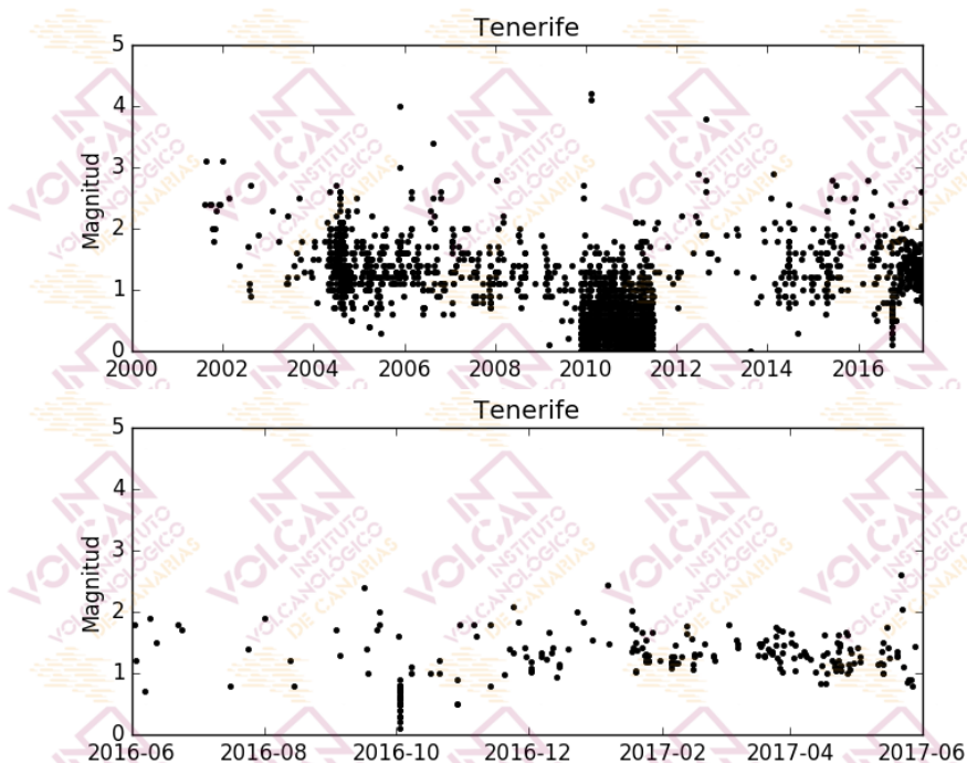
Figura 1.4 - Magnitudes de los terremotos localizados en el área de Tenerife. El gráfico superior corresponde al periodo enero 2000-mayo 2017, mientras que el inferior muestra el periodo junio 2016-mayo 2017. [La fuente de los datos sísmicos anteriores al 21/11/2016 es el Instituto Geográfico Nacional, IGN].
