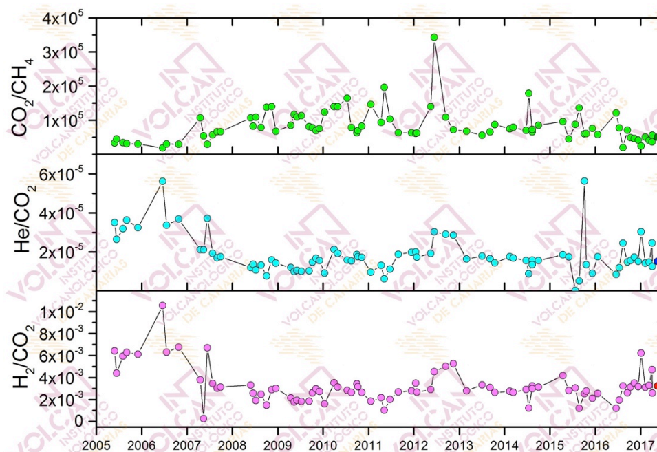
Figura 4.8 - Variaciones temporales de las relaciones molares \text{CO}_2/\text{CH}_4 , \text{He}/\text{CO}_2 y \text{H}_2/\text{CO}_2 en las fumarolas del Teide (TEF1). Los datos de mayo de 2017 se encuentran indicados en diferentes colores.
