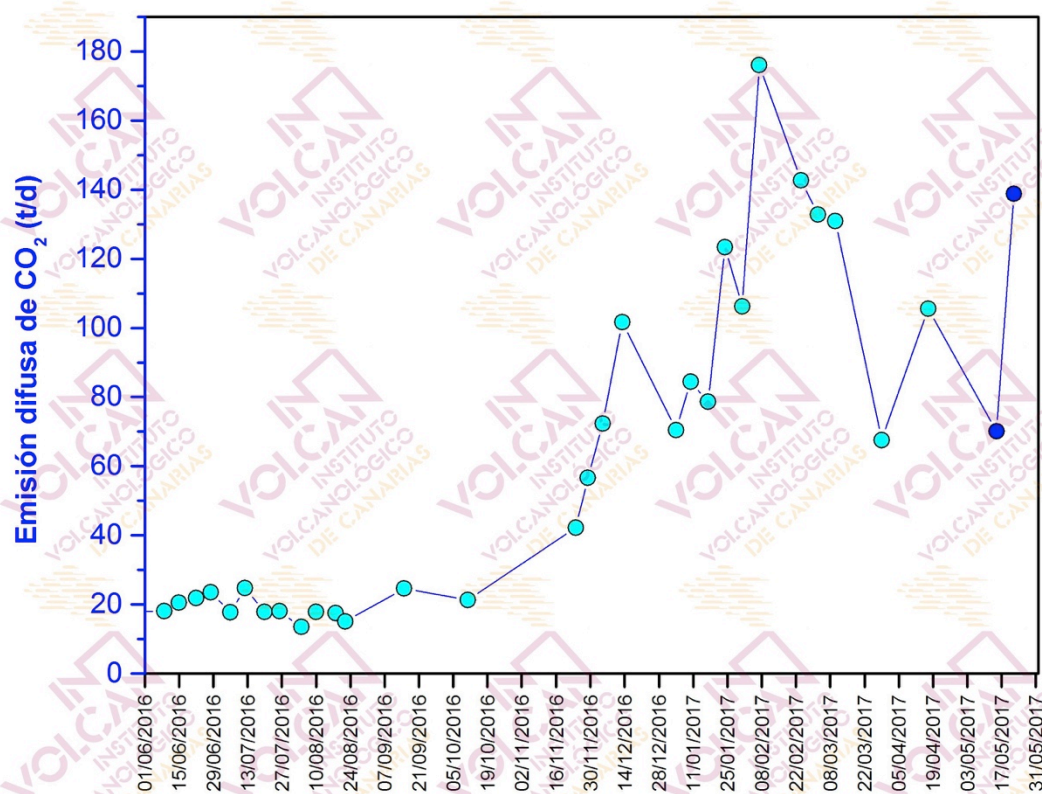
Figura 4.3 – Variaciones temporales de la emisión difusa de dióxido de carbono (CO 2 ) en el cráter del Teide durante los últimos 12 meses. Los datos de mayo de 2017 se encuentran marcados en azul oscuro.
