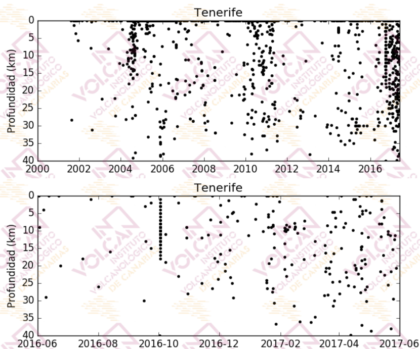
Figura 1.3 - Profundidades de los hipocentros localizados en el área de Tenerife. El gráfico superior corresponde al periodo enero 2000-mayo 2017, mientras que el inferior muestra el periodo junio 2016-mayo 2017. [La fuente de los datos sísmicos anteriores al 21/11/2016 es el Instituto Geográfico Nacional, IGN].
