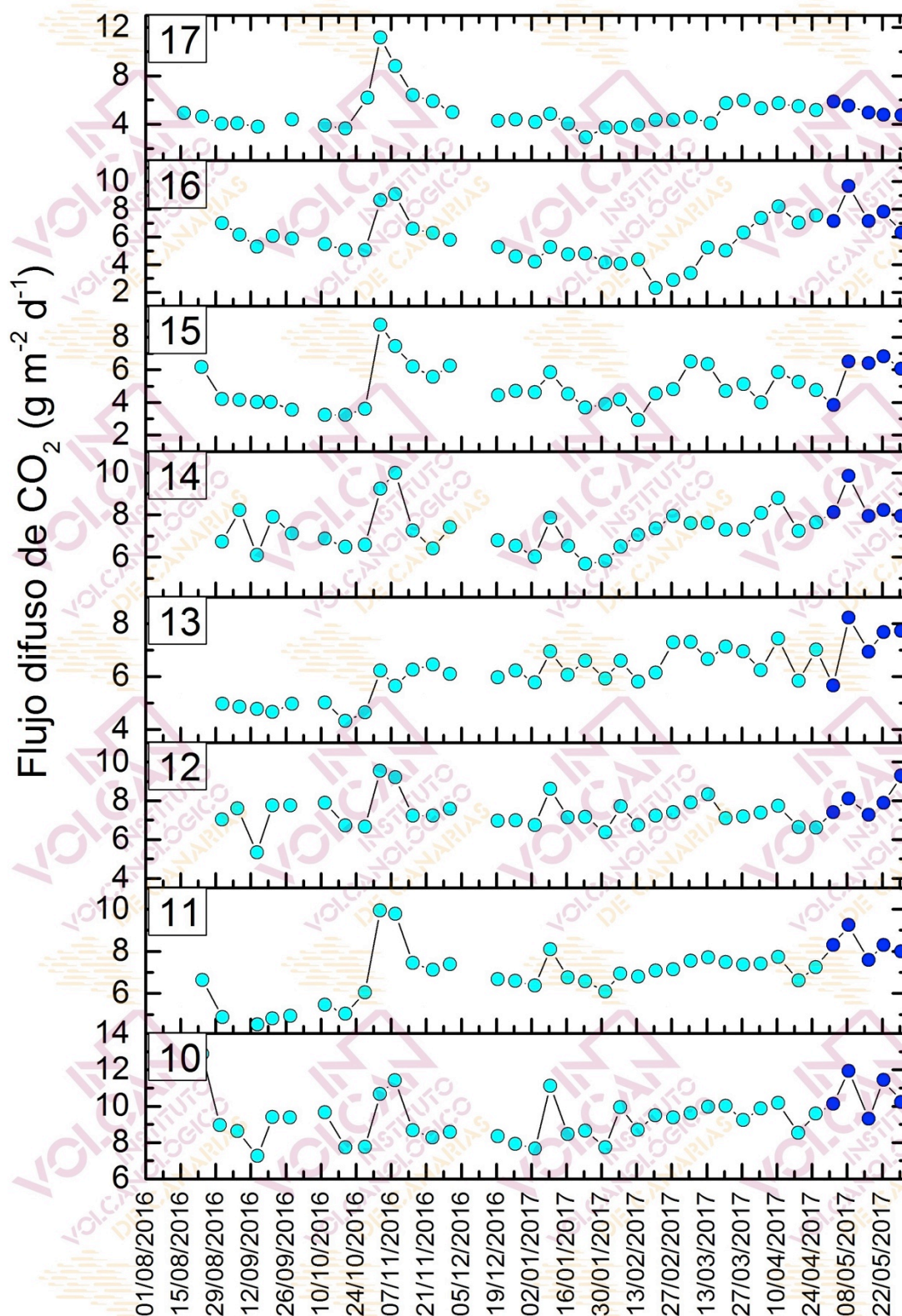
Figura 4.6 – Monitorización semanal del flujo difuso de CO 2 en la Red de Trampas Alcalinas del sistema volcánico Dorsal Norte-Sur de Tenerife desde agosto de 2016. Los datos de mayo de 2017 se encuentran marcados en azul oscuro.
