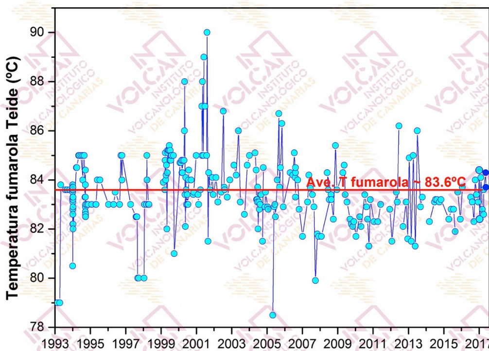
Figura 2.1 – Variaciones temporales de la temperatura registrada en la fumarola del Teide (TEF1) desde 1993. Los datos de mayo de 2017 se marcan en azul oscuro.
