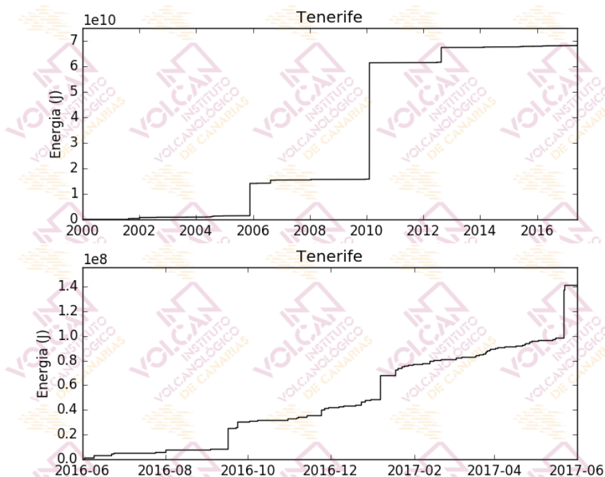
Figura 1.6 - Curva de energía sísmica acumulada por los terremotos localizados en el área de Tenerife. El gráfico superior corresponde al periodo enero 2000-mayo 2017, mientras que el inferior muestra el periodo junio 2016-mayo 2017. [La fuente de los datos sísmicos anteriores al 21/11/2016 es el Instituto Geográfico Nacional, IGN].
