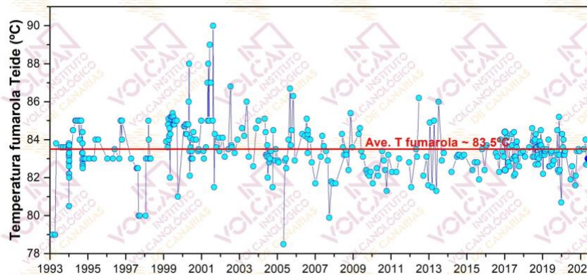
Figura 2.1 – Variaciones temporales de la temperatura registrada en las fumarolas del Teide (TEF1) desde 1993 hasta mayo 2021.
