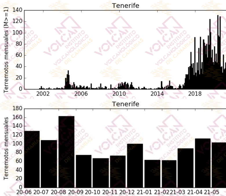
Figura 1.2 - Número de terremotos mensuales en Tenerife. El histograma superior corresponde al periodo enero 2000 – mayo 2021 para terremotos con M \geq 1 , mientras que el inferior muestra el periodo junio 2020 – mayo 2021 para todas las magnitudes. [La fuente de los datos sísmicos anteriores al 21/11/2016 es el Instituto Geográfico Nacional, IGN].
