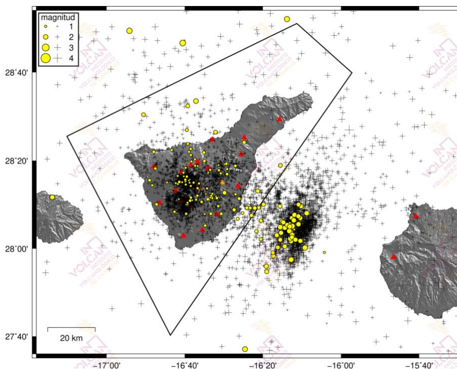
Figura 1.1 - Hipocentros de los terremotos (círculos amarillos) localizados por las estaciones de la Red Sísmica Canaria (triángulos rojos) en mayo de 2021. Las cruces muestran los hipocentros localizados en los últimos 12 meses. El polígono negro corresponde al área de Tenerife considerada en las estadísticas sismológicas de los gráficos siguientes.
