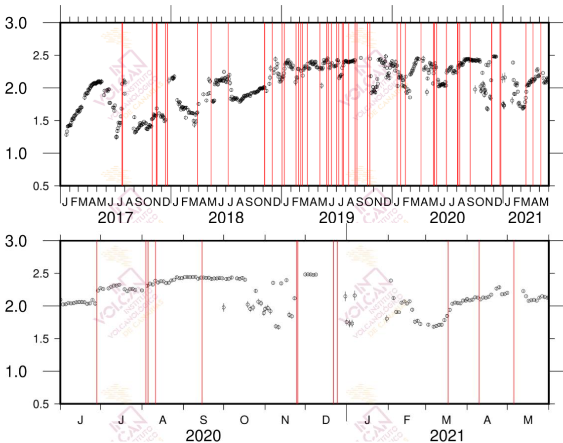
Figura 1.7 - Variaciones del parámetro b de la relación de Gutenberg-Richter. En el gráfico superior durante el periodo enero 2017 – mayo 2021. En el gráfico inferior durante el periodo junio 2020 – mayo 2021. Las líneas rojas indican la ocurrencia de enjambres sísmicos.
