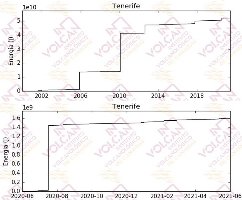
Figura 1.6 - Curva de energía sísmica acumulada por los terremotos localizados en el área de Tenerife. El gráfico superior corresponde al periodo enero 2000 – mayo 2021, mientras que el inferior muestra el periodo junio 2020 – mayo 2021. [La fuente de los datos sísmicos anteriores al 21/11/2016 es el Instituto Geográfico Nacional, IGN].
