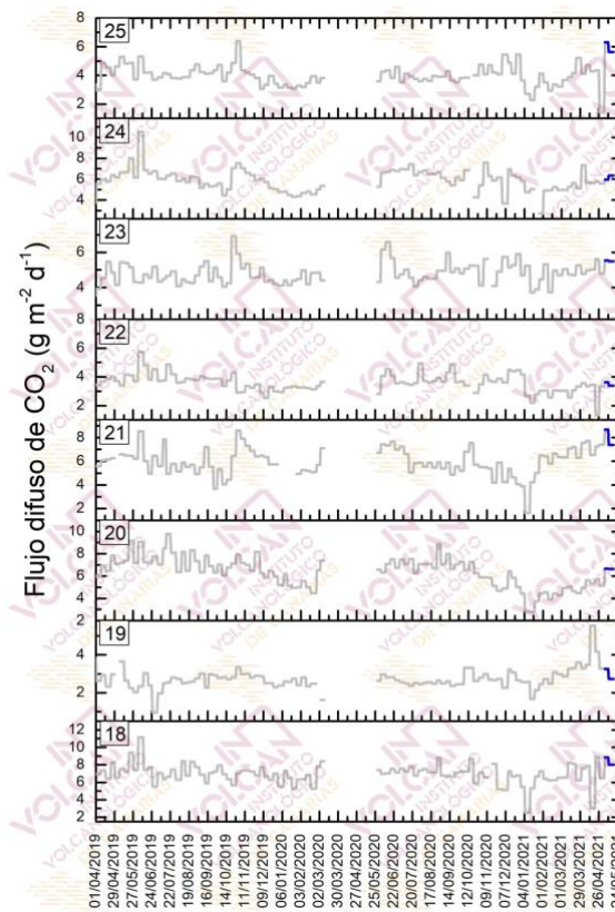
Figura 4.7 – Monitorización semanal del flujo difuso de CO 2 en la Red de Trampas Alcalinas de la Caldera de Las Cañadas desde junio de 2019. Los datos de mayo de 2021 se encuentran indicados en azul oscuro.
