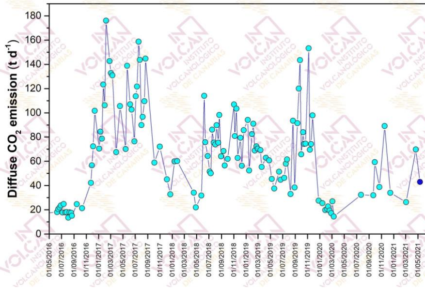
Figura 4.3 – Variaciones temporales de la emisión difusa de dióxido de carbono (CO 2 ) en el cráter del Teide desde el 1 de junio de 2016 hasta mayo 2021. Los datos de mayo de 2021 se encuentran indicados en azul oscuro.
