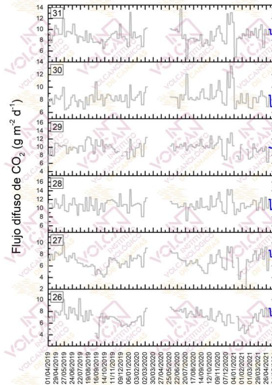
Figura 4.5 – Monitorización semanal del flujo difuso de CO 2 en la Red de Trampas Alcalinas del sistema volcánico Dorsal Noreste de Tenerife desde junio de 2019. Los datos de mayo de 2021 se encuentran indicados en azul oscuro.
