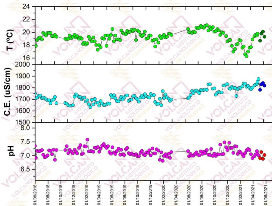
Figura 4.9 - Variaciones temporales de temperatura, conductividad ( \mu S \cdot cm^{-1} ) y pH medidas en el agua subterránea de la estación geoquímica TFG03. Los datos de mayo de 2021 se encuentran indicados en diferentes colores.
