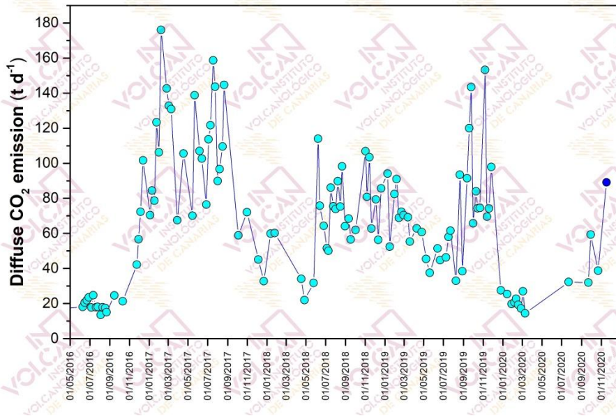
Figura 4.3 – Variaciones temporales de la emisión difusa de dióxido de carbono (CO 2 ) en el cráter del Teide desde el 1 de mayo de 2016.
