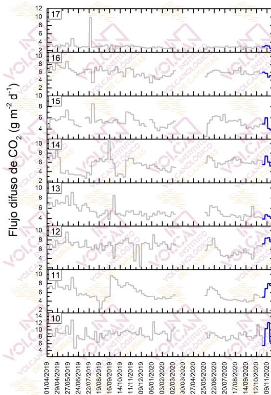
Tenerife desde abril de 2019. Los datos de noviembre de 2020 se encuentran indicados en azul oscuro.
