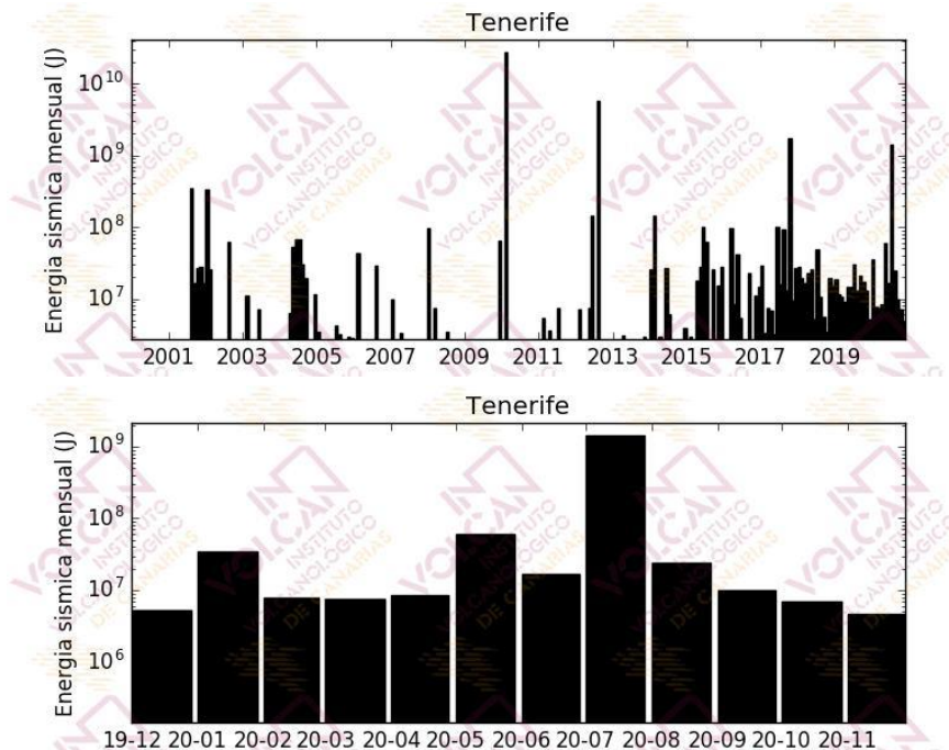
Figura 1.5 – Energía sísmica liberada por los terremotos localizados en el área de Tenerife. El histograma superior corresponde al periodo enero 2000 – noviembre 2020, mientras que el inferior muestra el periodo diciembre 2019 – noviembre 2020. [La fuente de los datos sísmicos anteriores al 21/11/2016 es el Instituto Geográfico Nacional].
