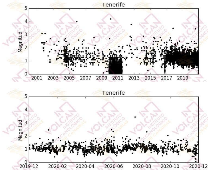
Figura 1.4 - Magnitudes de los terremotos localizados en el área de Tenerife. El gráfico superior corresponde al periodo enero 2000 – noviembre 2020, mientras que el inferior muestra el periodo diciembre 2019 – noviembre 2020. [La fuente de los datos sísmicos anteriores al 21/11/2016 es el Instituto Geográfico Nacional, IGN].
