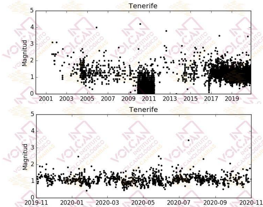
Figura 1.4 - Magnitudes de los terremotos localizados en el área de Tenerife. El gráfico superior corresponde al periodo enero 2000 – octubre 2020, mientras que el inferior muestra el periodo noviembre 2019 – octubre 2020. [La fuente de los datos sísmicos anteriores al 21/11/2016 es el Instituto Geográfico Nacional, IGN].
