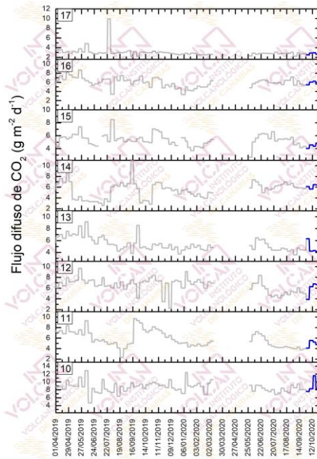
Figura 4.7 – Monitorización semanal del flujo difuso de CO 2 en la Red de Trampas Alcalinas de la Caldera de Las Cañadas desde abril de 2019. Los datos de octubre de 2020 se encuentran indicados en azul oscuro.
