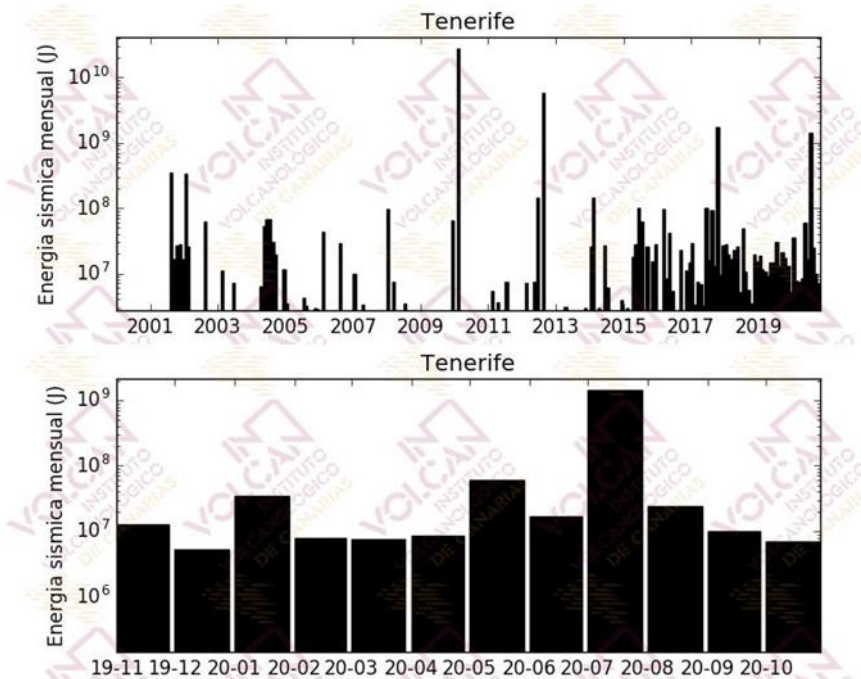
Figura 1.5 – Energía sísmica liberada por los terremotos localizados en el área de Tenerife. El histograma superior corresponde al periodo enero 2000 – octubre 2020, mientras que el inferior muestra el periodo noviembre 2019 – octubre 2020. [La fuente de los datos sísmicos anteriores al 21/11/2016 es el Instituto Geográfico Nacional].
