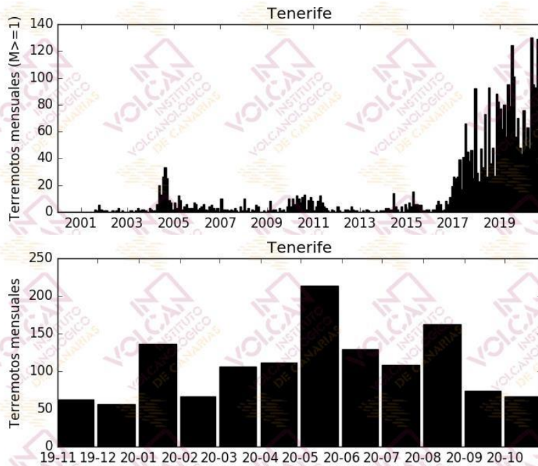
Figura 1.2 - Número de terremotos mensuales en Tenerife. El histograma superior corresponde al periodo enero 2000 – octubre 2020 para terremotos con M \geq 1 , mientras que el inferior muestra el periodo noviembre 2019 – octubre 2020 para todas las magnitudes. [La fuente de los datos sísmicos anteriores al 21/11/2016 es el Instituto Geográfico Nacional, IGN].
